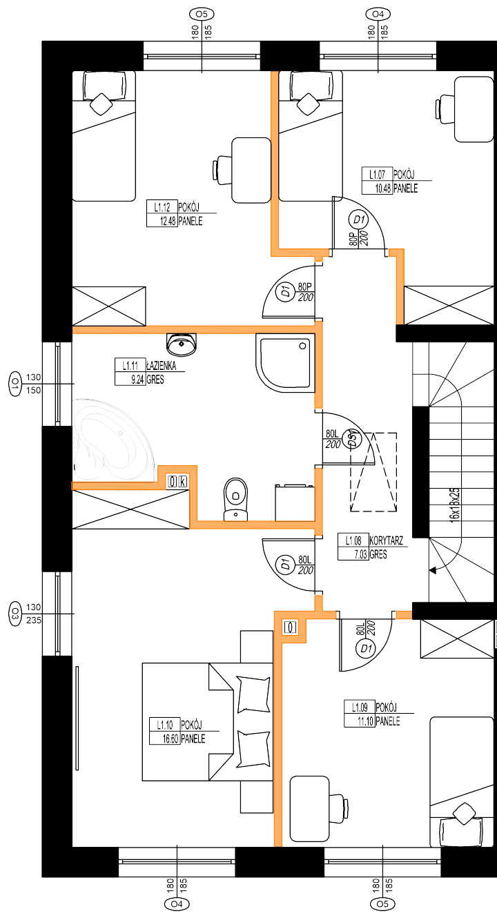
RZUT PIĘTRA
